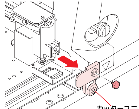
カッターユニット
